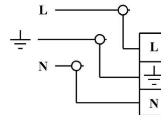
Рис1. Схема подключения светильника.
